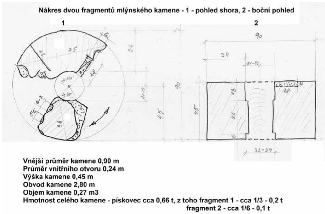
Obr. Nákres s parametry obou částí mlýnského mlecího kamene.
